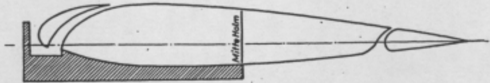
Arbeitslehre für Vorflügel bei Rippe 4 anlegen
