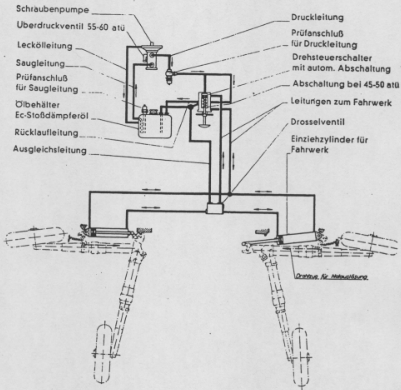
Drehsteuerschalter
