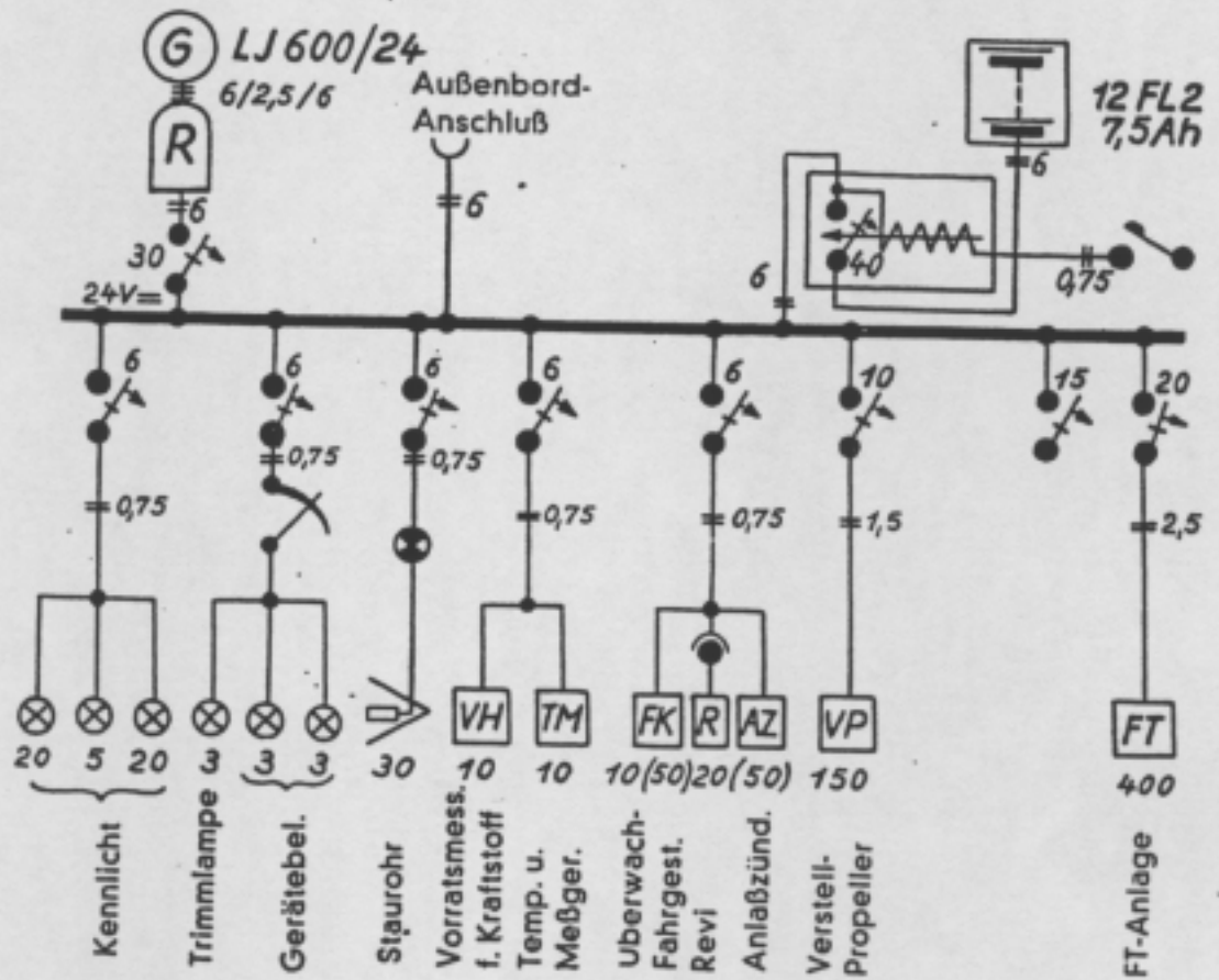
Schaltplan
