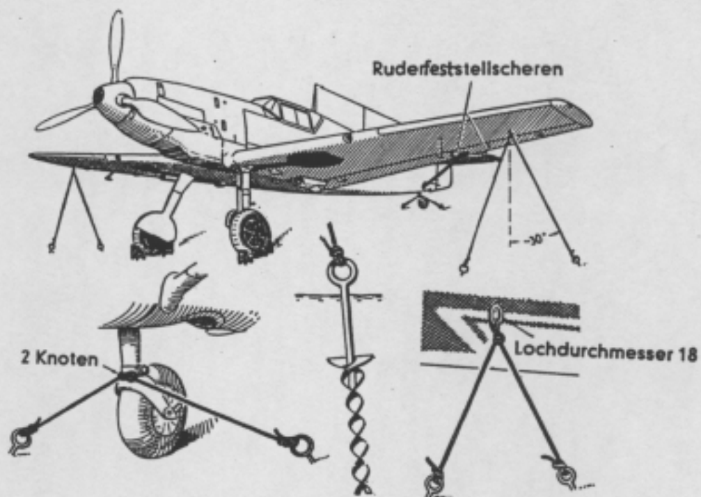
Verankerungsplan
