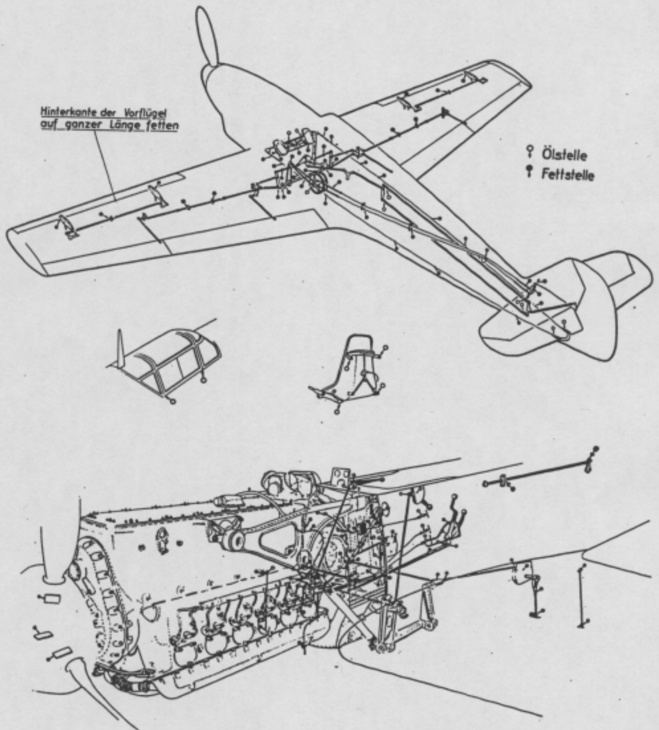
Schmierplan für Steuerung und Triebwerk
