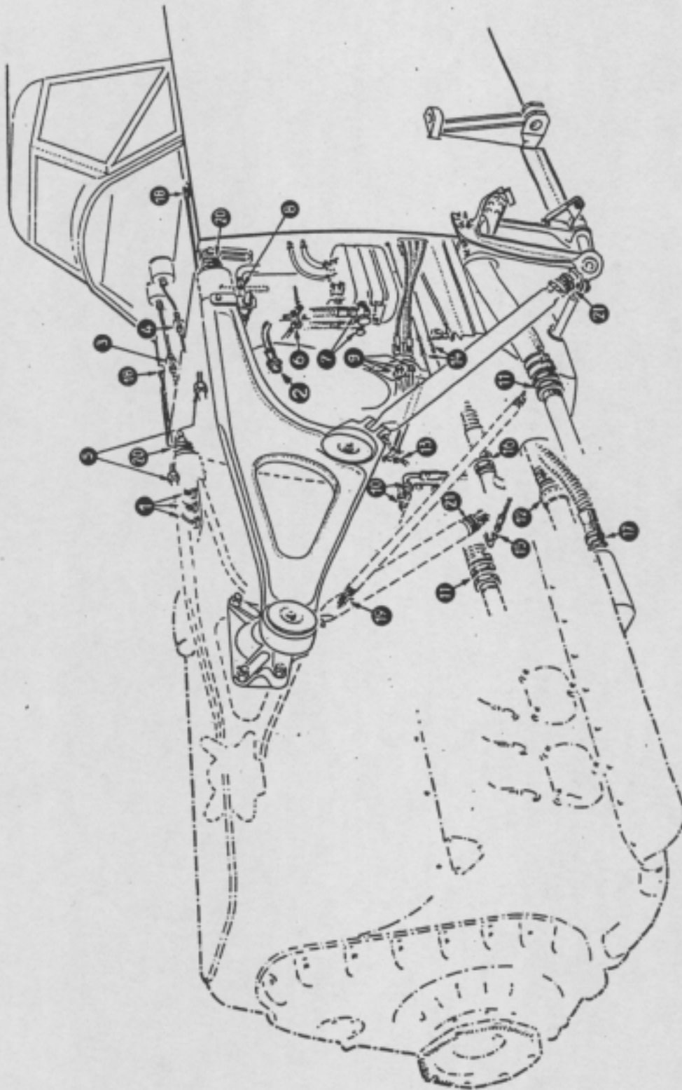
Trennstellen für Triebwerkswechsel
