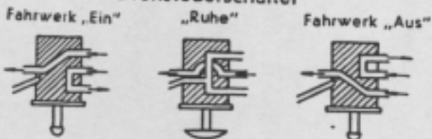
Drehsteuerschalter
